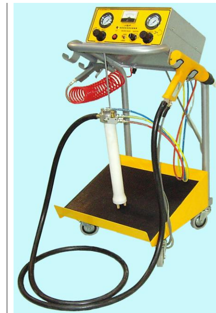
APARATI ZA TRANSPORT I NANOŠENJE PRAHOVA
